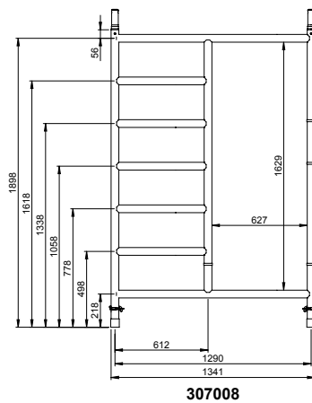
Durchstiegsrahmen RS TOWER 52
