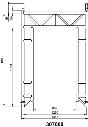
Basis-Durchstiegsrahmen RS TOWER 52
