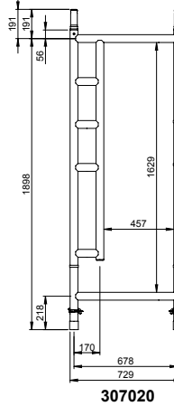
Durchstiegsrahmen RS TOWER 51
